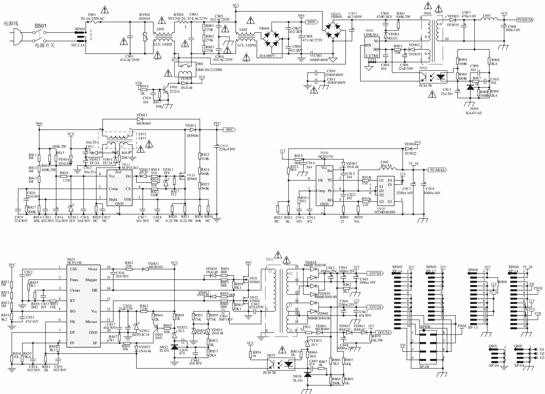
海信液晶TLM40V68P (2) 系列 (1673板) 电视接收机电源电路原理图
